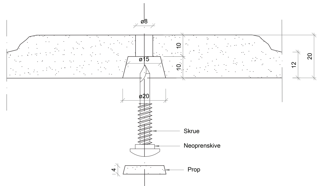
Montage detalje, 1:1 Prop monteres med limende fugemasse.
